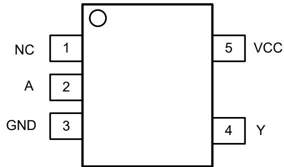
SOT23-5/SC70-5
